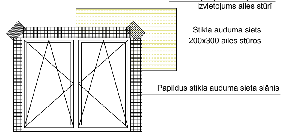
Isolācijas ierīkošana ap logu aili
